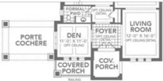
ELEVATION B
